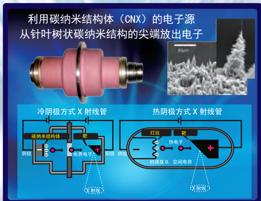
冷阴极X射线管
