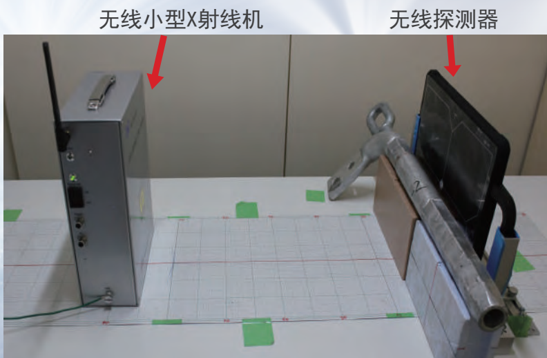
检测实景
