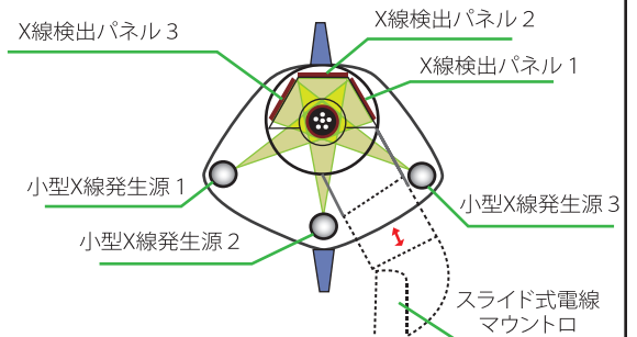
3 方向原理図
